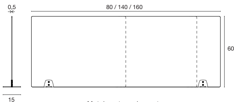
Metalen steunelement
