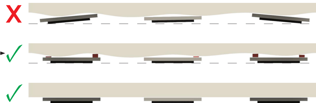
Abbildung 1 - Draufsicht -
